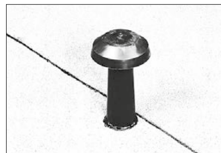
Fot. 2. Po zgrzaniu sąsiedniego brytu papę podstawę kominka należy uszczelnić uszczelnianiem bitumicznym oraz zamontować czaszę kominka na szczycie tubusu.
