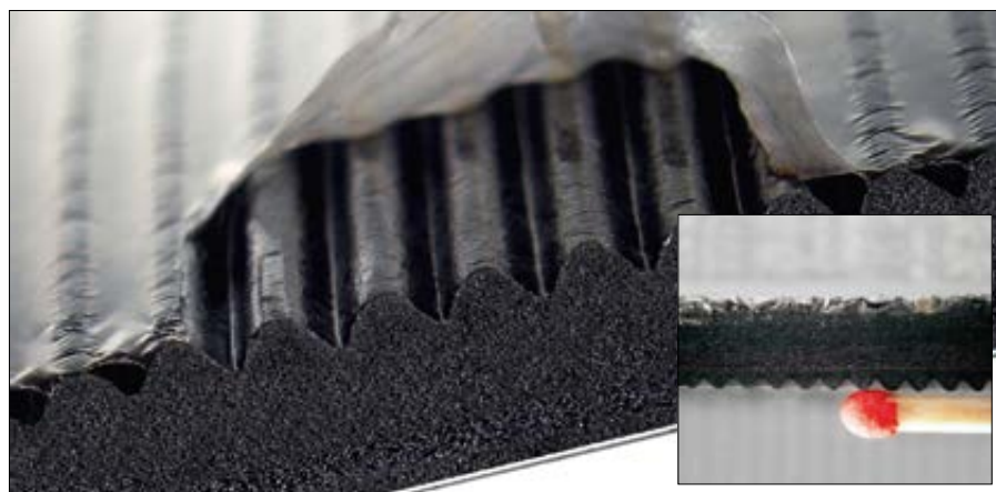
Rys. 2. Profilowana budowa spodniej części papy zapewnia bardziej efektywne wytapianie asfaltu.
