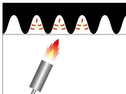
Rys. 2. Profilowana budowa spodniej części papy zapewnia bardziej efektywne wytapianie asfaltu.
