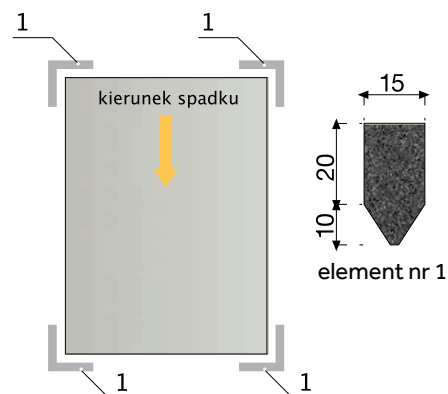
Pokrycie połaci z papy podkładowej
