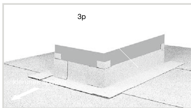
Pokrycie połaci z papy podkładowej
