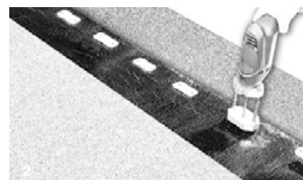
2. Rozmieszczenie łączników przy mocowaniu papy do jednowarstwowych pokryć dachowych mocowanych mechanicznie MONODACH WM lub MONOLight.
